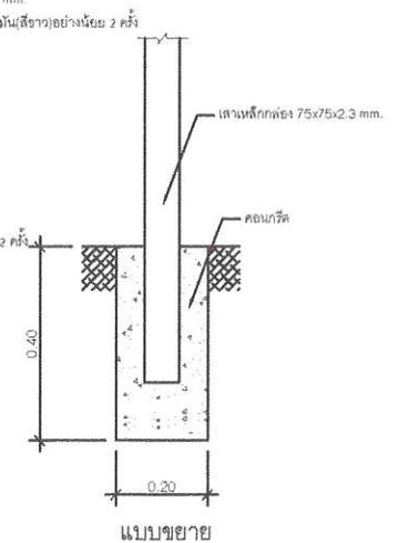
แบบขยาย
