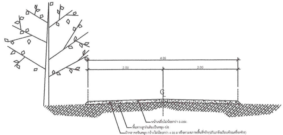
แบบรูปตัด A มาตราส่วน 1 : 50
