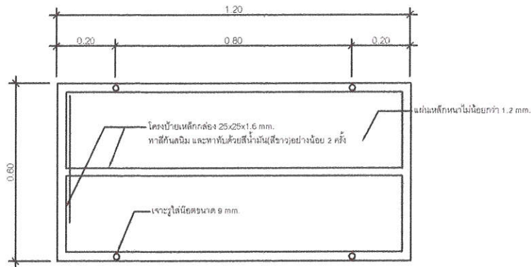
รูปป้ายด้านหลัง
