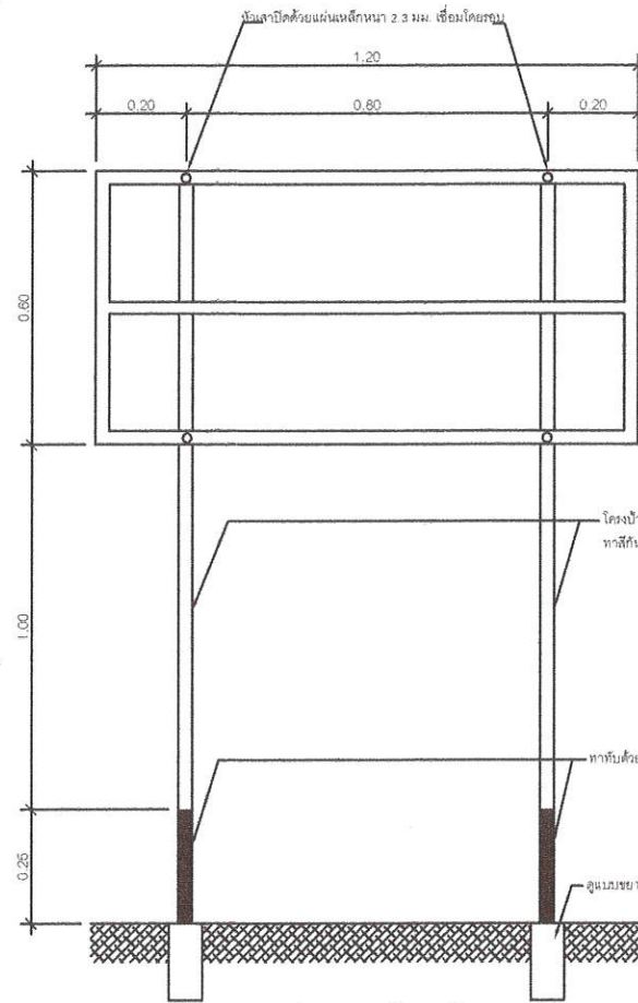
รูปแสดงการปักเสาป้าย
