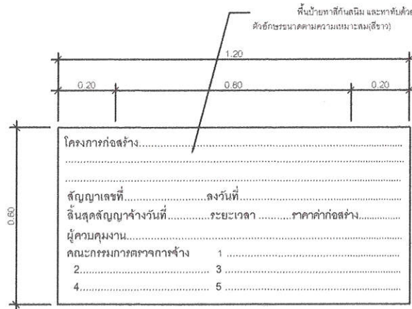
รูปป้ายด้านหน้า
