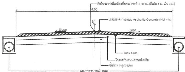
รูปตัดตามขวางงานฉาบผิว Asphaltic Concrete (Hot mix) NOT TO SCALE
