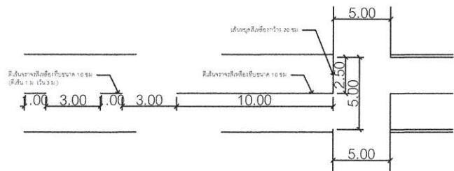
รูปขยายงานตีเส้นจราจร NOT TO SCALE
